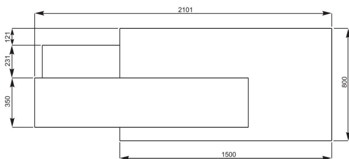
Draufsicht
