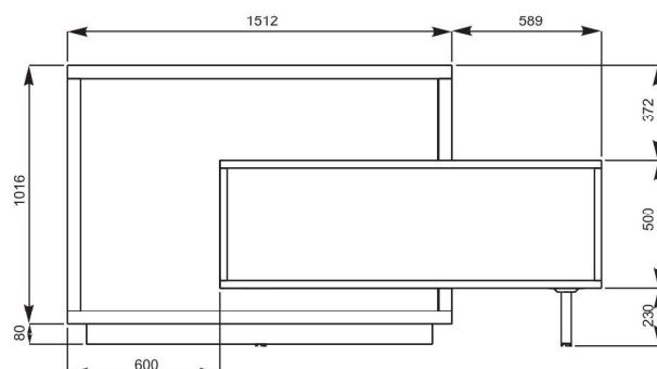
Ansicht Front
